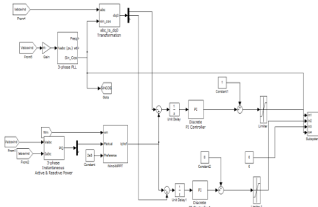
Fig 10. PMSG controller
